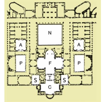
Grundriss der Trajansthermen in Rom
